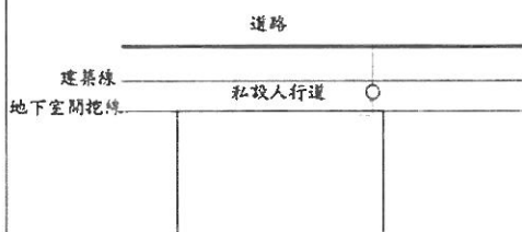
圖1-4 建築物表位設於私設人行道
