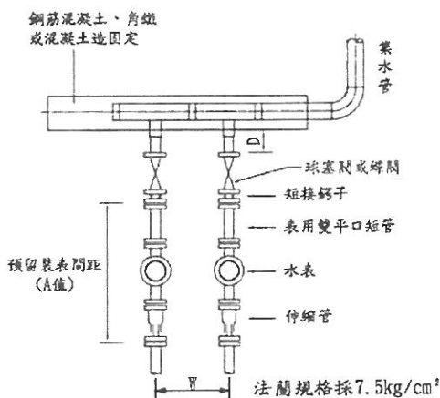
圖4-2 大表分表表位裝置圖
