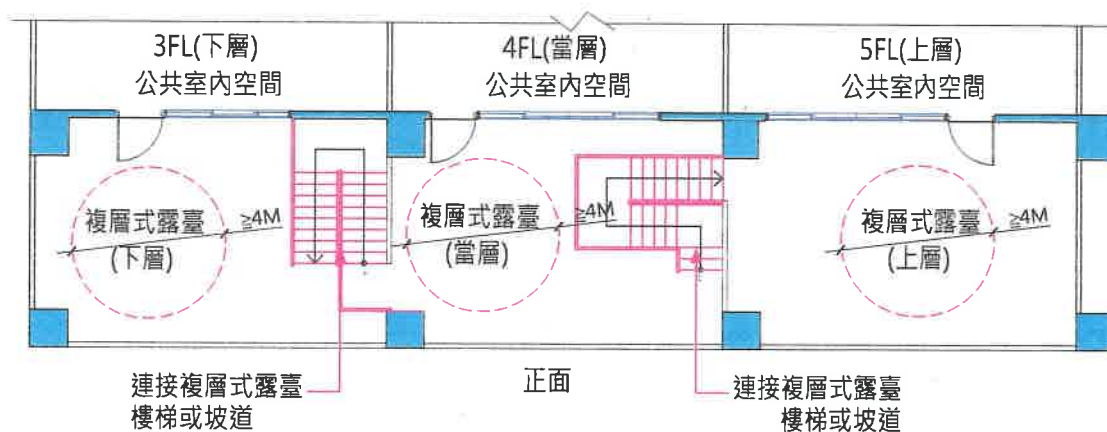
平面圖
